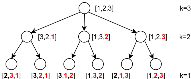
Slika 6.7: Rekurzivno generisanje permutacija niza 123 korišćenjem razmena elemenata niza
