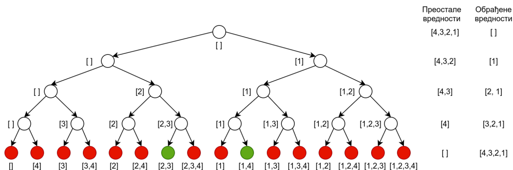
Slika 7.4: Gruba sila – ispitivanje svih podnizova
