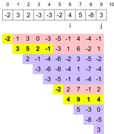
Slika 3.2: Maksimalni zbir segmenta. Žutom bojom su obeleženi zbrojevi koji se proveravaju, crvenom oni koji se mogu preskočiti jer im prethodni negativni zbir, a plavom oni koji se mogu preskočiti jer se iznad početka njihove vrste nalazi pozitivan zbir.
