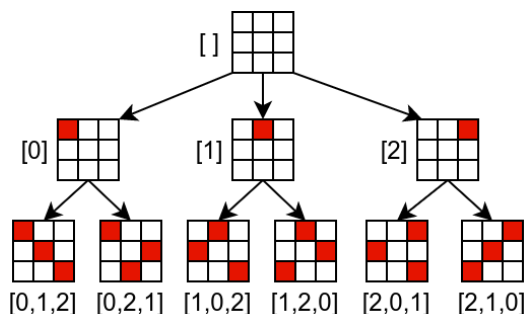
Slika 7.2: Raspoređivanje 3 dame – sve permutacije i pozicije koje su njima predstavljene
