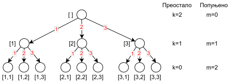
Slika 6.3: Rekurzivni postupak generisanja varijacija dužine 2 od elemenata skupa {1, 2, 3}
