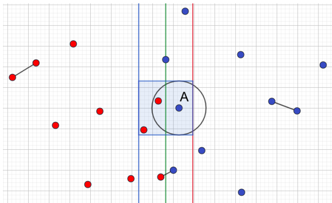
Slika 5.2: Najbliži par tačaka u levom pojasu, desnom pojasu i između pojaseva. Krug i kvadrat koji sadrže tačke koje se porede sa tačkom A .
