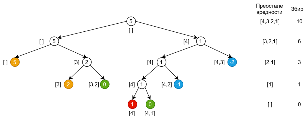
Slika 7.9: Pretraga sa odsecanjem
