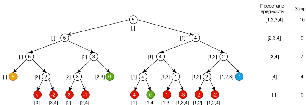
Slika 7.6: Pretraga uz osnovno odsecanje
