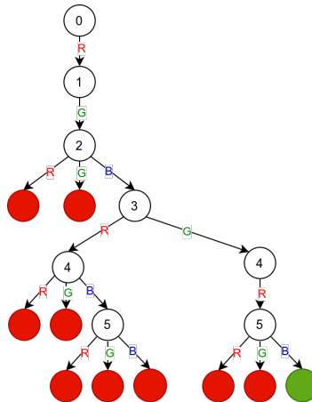
Slika 7.11: Drvo pretrage pridruženom bojenju grafa sa 3 boje
