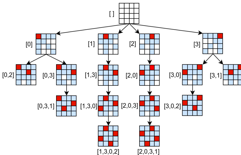
Slika 7.3: Raspoređivanje 4 dame - pretraga sa odsecanjem
