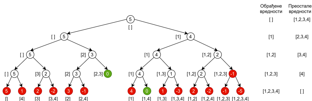
Slika 7.5: Gruba sila – preostali ciljni zbir
