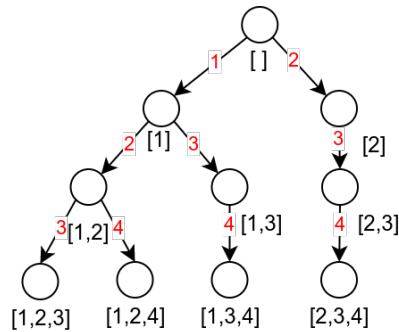
Slika 6.4: Rekurzivno generisanje kombinacija dužine 3 iz skupa {1, 2, 3, 4}
