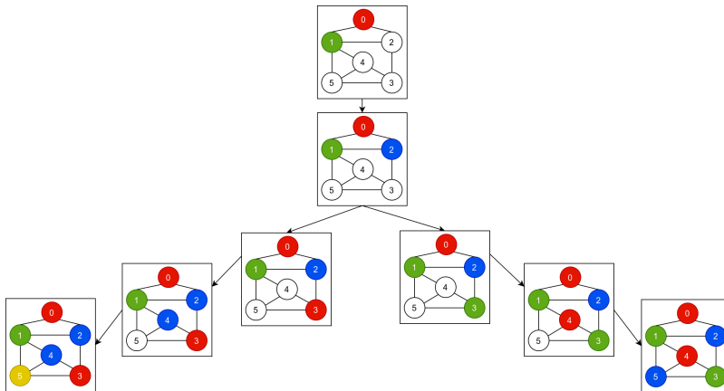
Slika 7.12: Primer bojenja grafa sa minimalnim brojem boja
