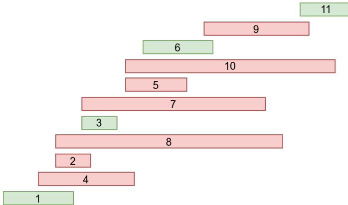
Slika 9.10: Rezultat primene dualne gramzive strategije
