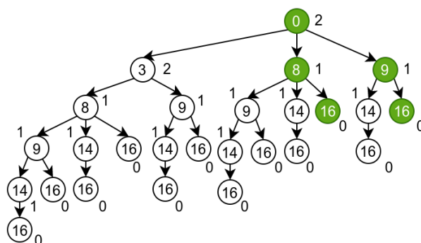
Slika 9.3: Drvo iscrpne pretrage
