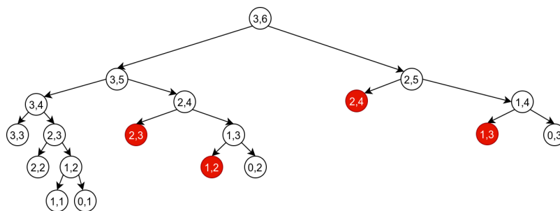
Slika 8.3: Drvo rekurzivnih poziva uz memoizaciju
