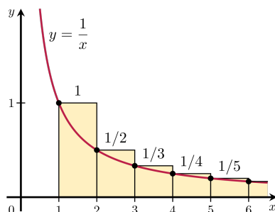
Slika 2.12: Procena zbira harmonijskog reda H(n) određenim integralom
