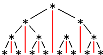
Slika 2.7: Broj čvorova na najnižem nivou binarnog drveta za jedan je veći od ukupnog broja čvorova na prethodnim nivoima
