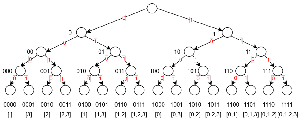
Slika 6.2: Svi podskupovi četvoročlanog skupa - svaki list drveta odgovara jednom podskupu
