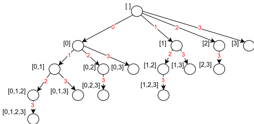
Slika 6.1: Svi podskupovi četvoročlanog skupa - svaki čvor drveta odgovara jednom podskupu
