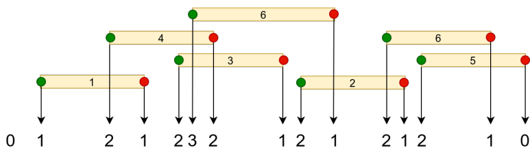
Slika 9.7: Obilazak svih karakterističnih tačaka uz ažuriranje brojača
