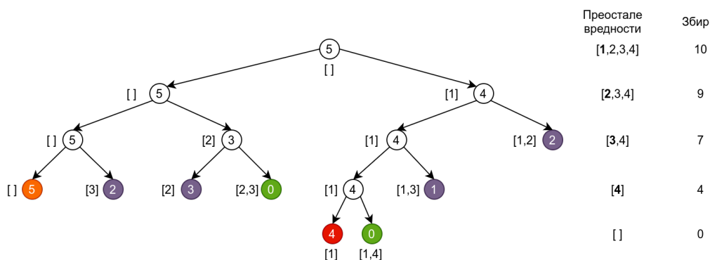
Slika 7.8: Pretraga sa odsecanjem
