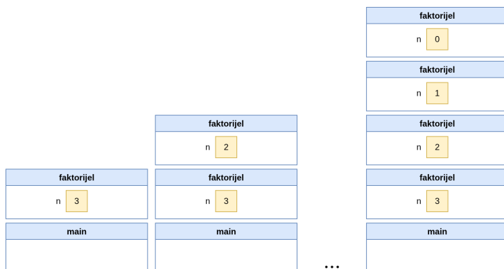
Slika 4.1: Stek okviri prilikom poziva faktorijel(3)
