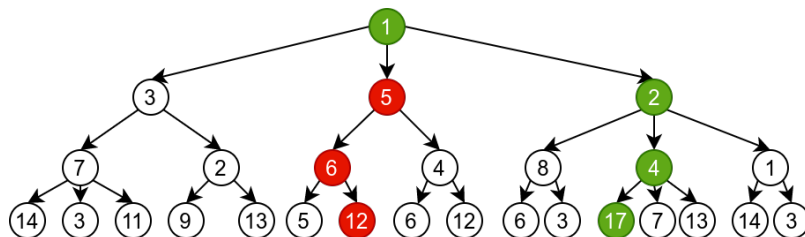
Slika 9.2: Drvo pretrage kod kojeg pohlepni algoritam ne dovodi do optimalnog rešenja tj. rešenja maksimalne vrednosti
