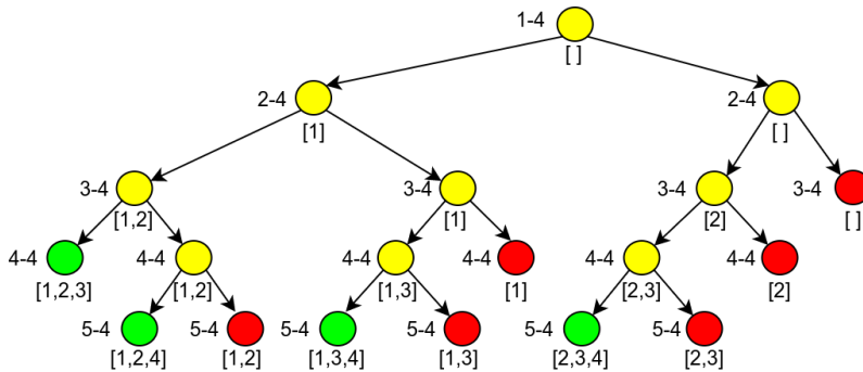
Slika 6.5: Rekurzivno generisanje kombinacija - levo od svakog čvora je prikazan raspon preostalih vrednosti, ispod čvora tekuća kombinacija. U zelenim čvorovima su uspešno generisane kombinacije, a u crvenim nastupa odsecanje, jer raspon ne sadrži dovoljno vrednosti da bi se kombinacija generisala do kraja
