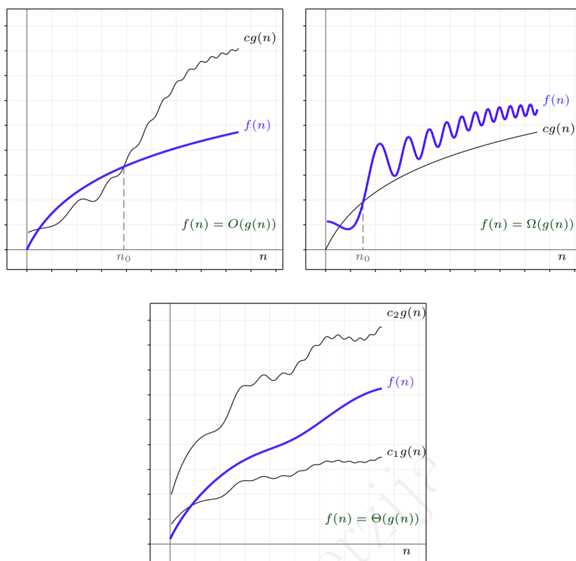
Slika 2.3: Ilustracija pojmova “veliko o”, “veliko omega” i “veliko teta”
