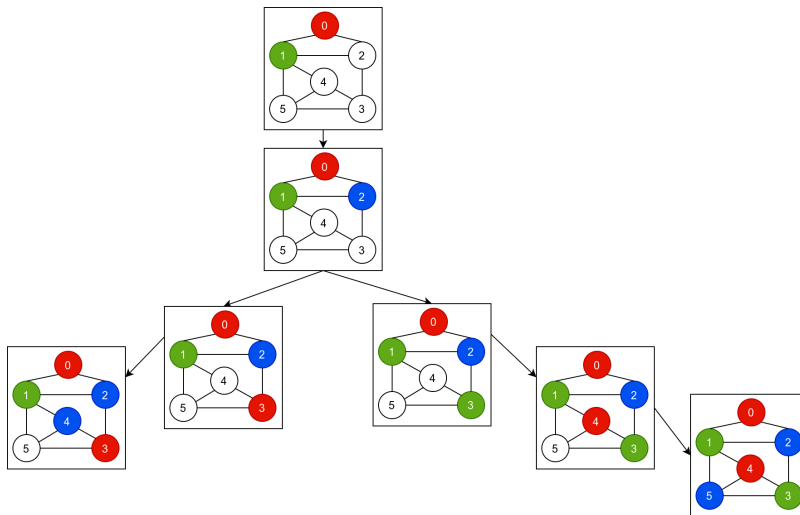
Slika 7.10: Primer bojenja grafa sa 3 boje
