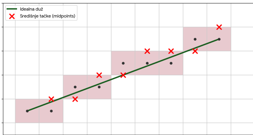
Slika 3.3: Bresenhamov algoritam
