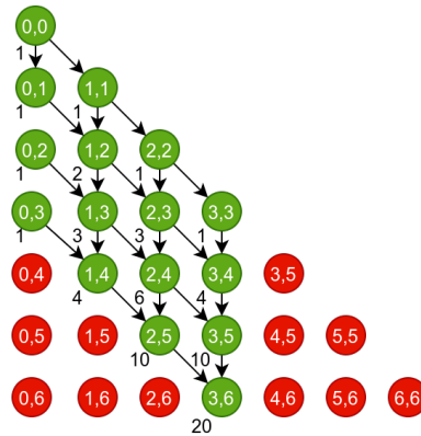
Slika 8.4: Elementi Paskalovog trougla potrebni za izračunavanje broja \binom{6}{3}
