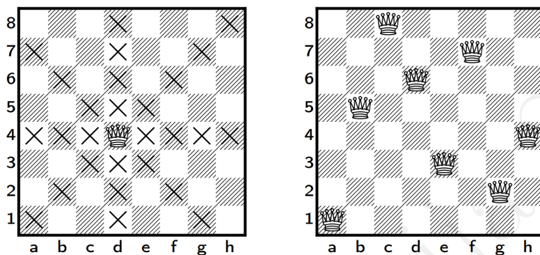
Slika 7.1: Problem 8 dama
