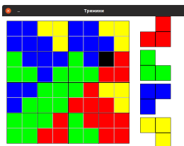
Slika 5.1: Trimini
