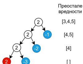
Slika 7.7: Doprinos odsecanja na osnovu vrednosti najmanjega elementa
