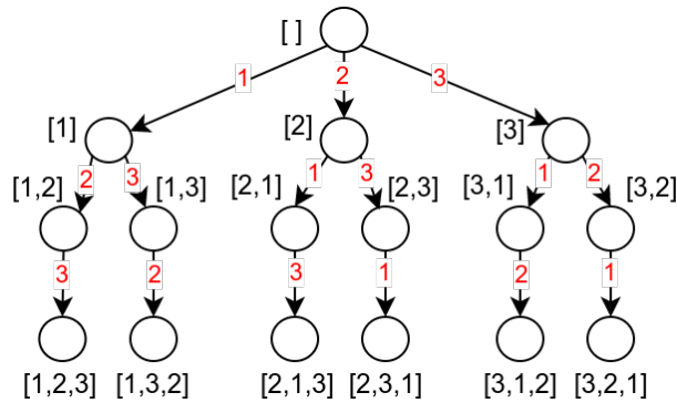
Slika 6.6: Rekurzivno generisanje permutacija niza 123 - na tekuću poziciju se postavlja jedan po jedan element niza 123, koji nije već postavljen na prethodne pozicije
