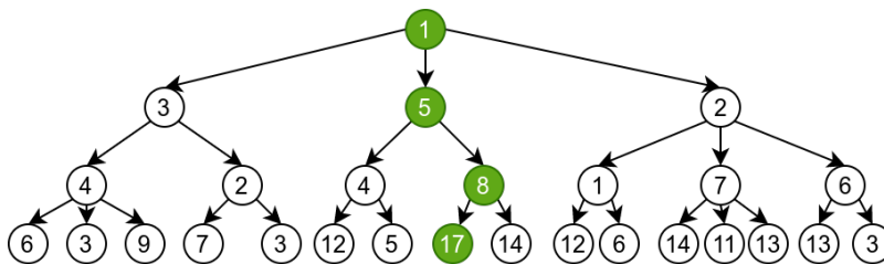
Slika 9.1: Drvo pretrage kod kojeg pohlepni algoritam dovodi do optimalnog rešenja tj. rešenja maksimalne vrednosti
